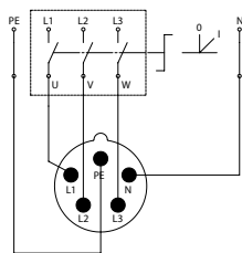
Rozłącznik 0-I
