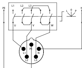
Przełącznik L-0-P
